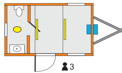
4 08X16' OFICINA C/BAÑO EXT. 2.44X4.88 INT. 2.26X3.48
