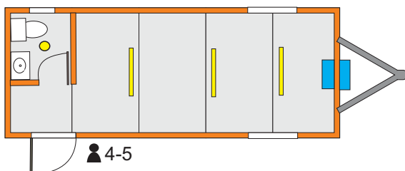
8 08X24' OFICINA C/BAÑO EXT. 2.44X7.32 INT. 2.26X5.92m
