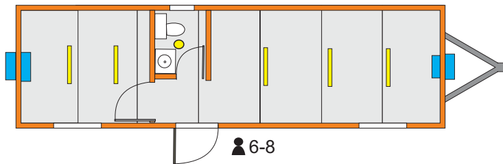
9 08X32' OFICINA C/BAÑO Y UN PRIVADO EXT. 2.44X9.76 INT. 2.26X8.36m
