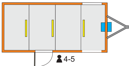
5 08X20' OFICINA EXT. 2.44X6.10 INT. 2.26X4.70m
