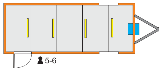
7 08X24' OFICINA EXT. 2.44X7.32 INT. 2.26X5.92m
